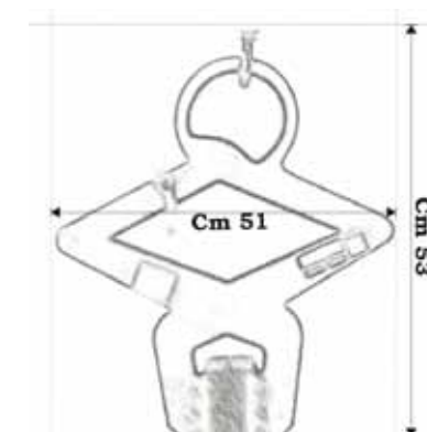
DIMENSIONI PINZA IN POSIZIONE CHIUSA CLAMP DIMENSIONS WHEN CLOSE
