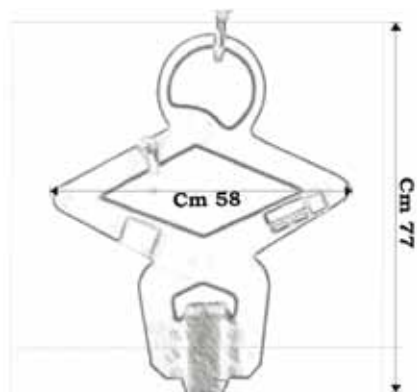
DIMENSIONI PINZA IN POSIZIONE CHIUSA CLAMP DIMENSIONS WHEN CLOSE
